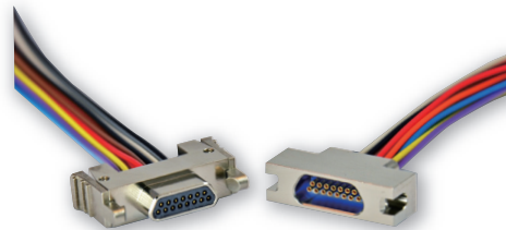
〈0.635mm,1.27mmピッチコネクタ〉
