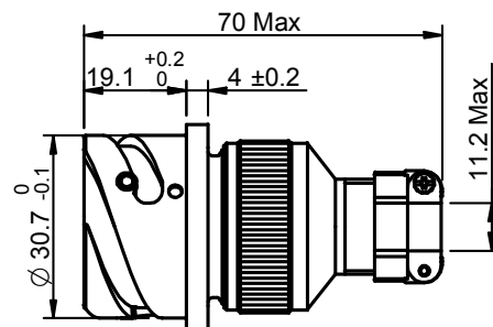
FRITS0018-USBA-1N1F6
