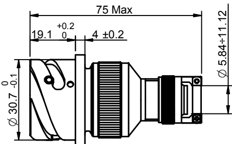
FRITS0018-USBA-1N5F6
