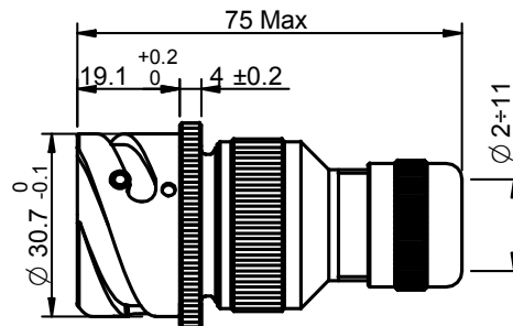
FRITS0118-USBA-1PHMF6
