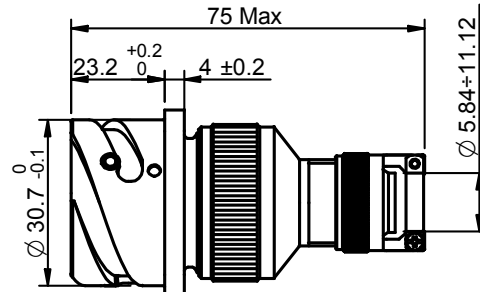
FRITS03018-USBA-1N5F6
