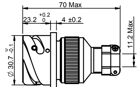
FRITS03018-USBA-1N1F6
