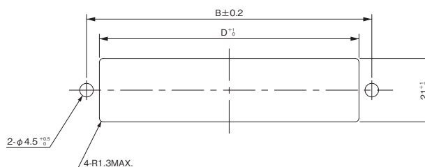
パネル取付穴寸法(参考)
