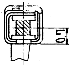
ピン挿入図
