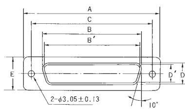
結合後の寸法
