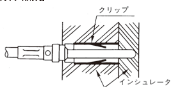
①引抜工具挿入
