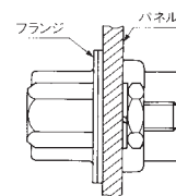
フロントマウント
