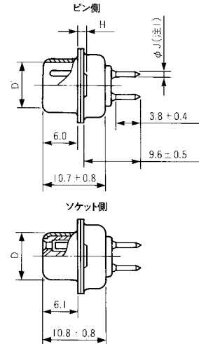
(注1) 端末形状
