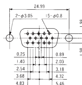
基板取付穴寸法
