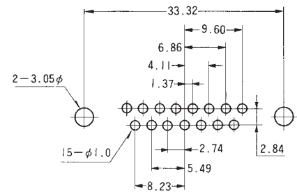
DA-15
