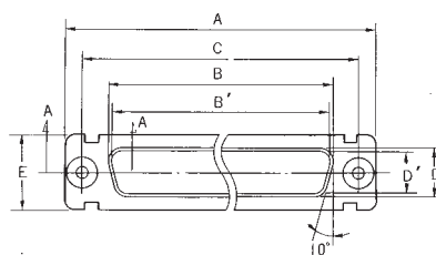
フローティング部 (A-A)
