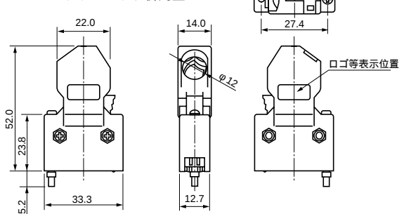
ジャックソケットスクリューL26型
