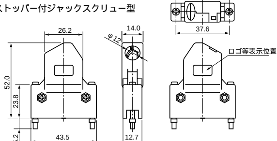
ストッパー付ジャックスクリュー型
