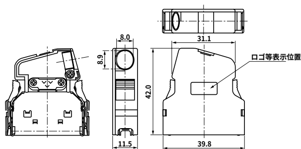
36極の場合
